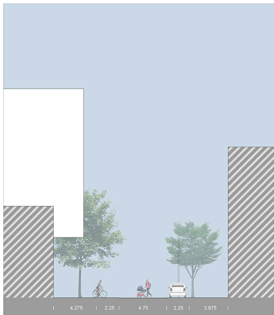
B-Straße Querschnitt
