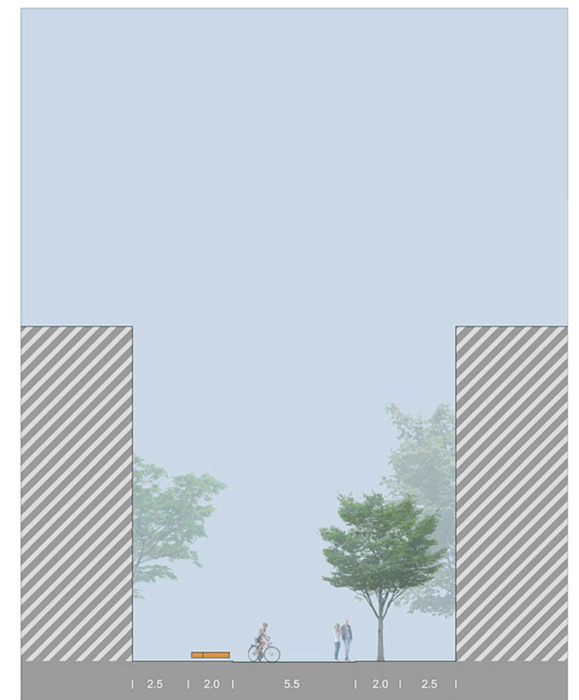
C-Straße Querschnitt
